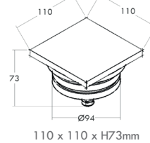
110 x 110 x H73mm
